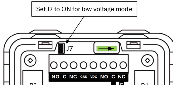
Fig. 14. Low lock voltage
